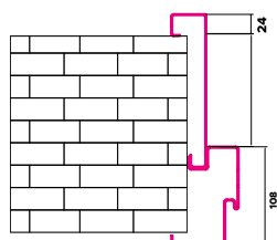
Opaska z ościeżnicą regulowaną IRON
